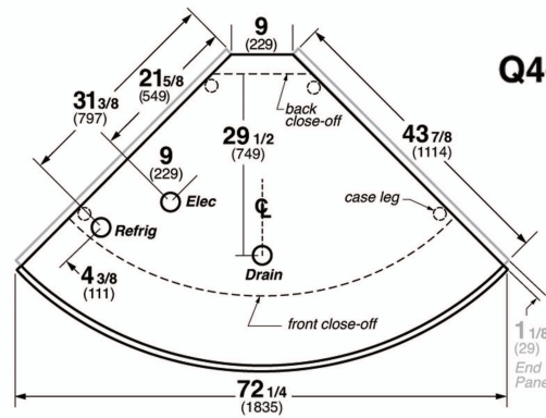
Q4-SS 45° O/S wedge
