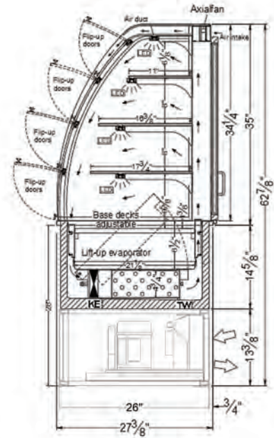
VICD(A)-34-R-CV-SC FD
