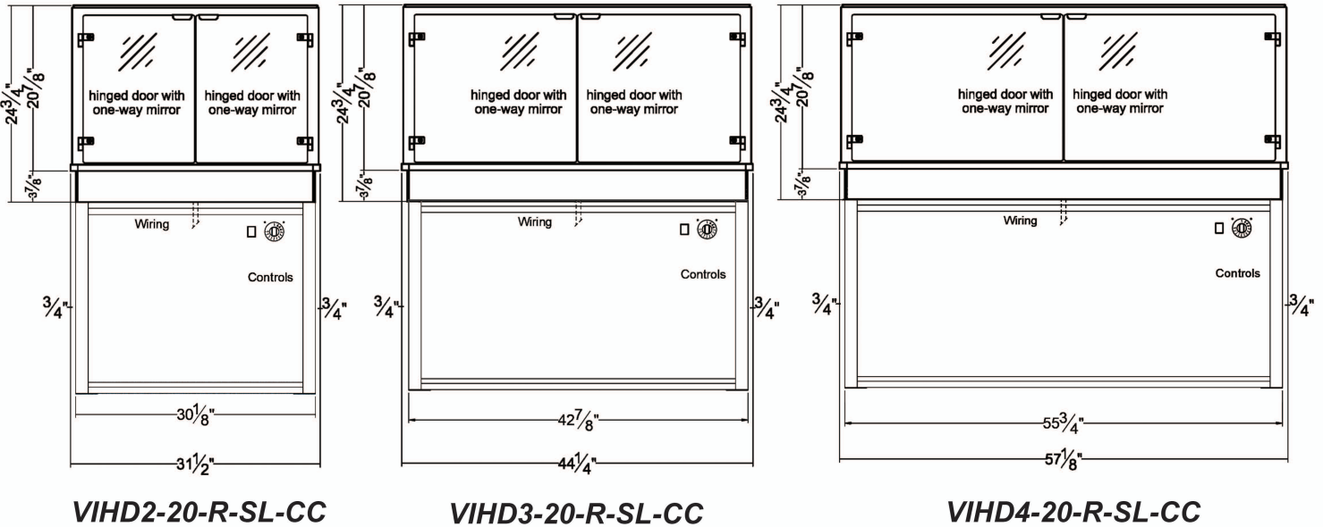
VIHD(A)-20-R-SL-CC
