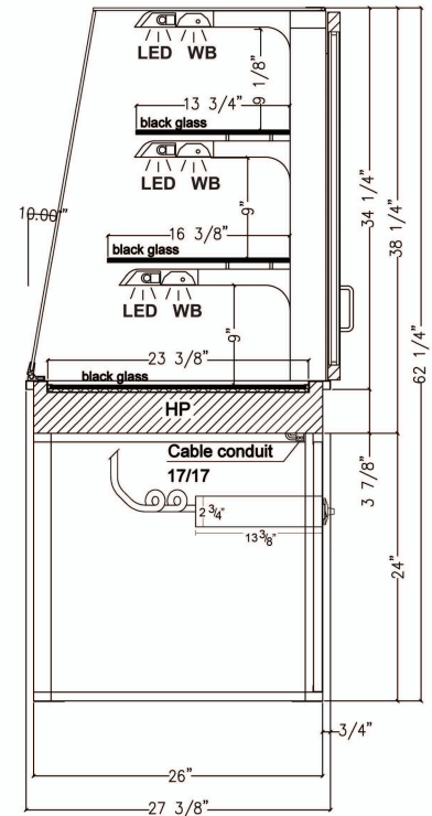
VIHD(A)-34-R-SL-CC
