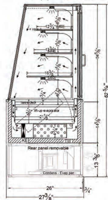
VICD(A)-34-R-SL-SC INS
